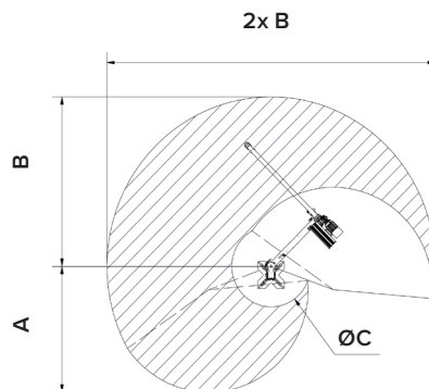
Högerhängd Mobichain
