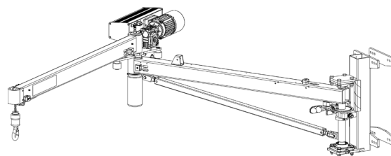
Väggmonterad kran
