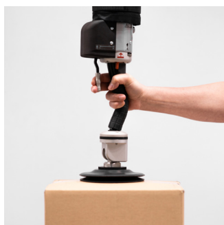
Bälsugkopp ø150, ø200
